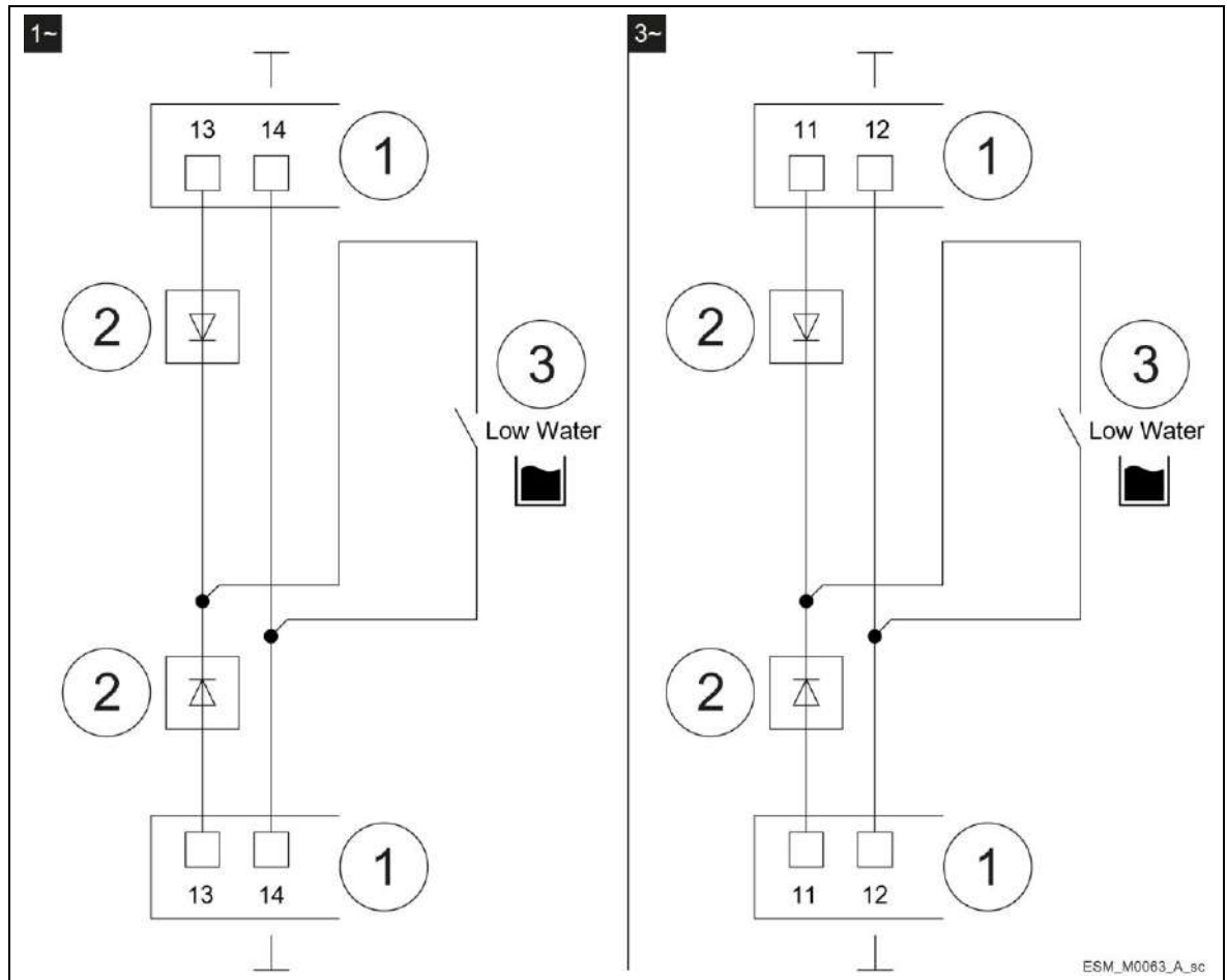
Figura 12: Diodo
