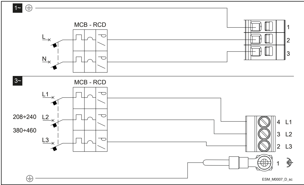
Figura 9: Diagrama de cableado
