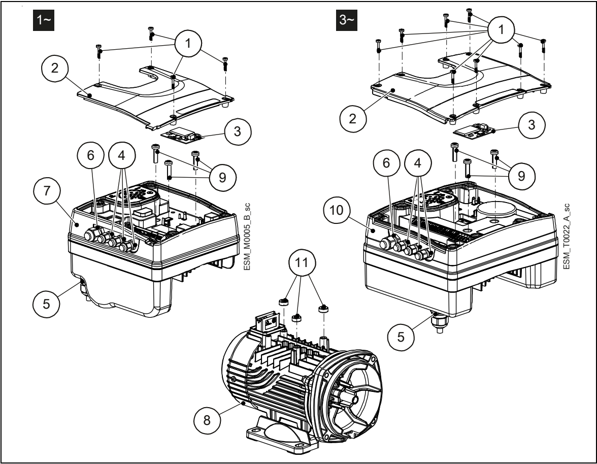
Figura 6: Componentes principales - Modelos monofásico y trifásico
